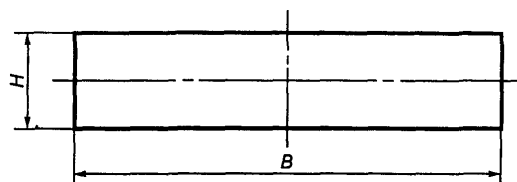
Рисунок Д.6. Размеры знаков 1.34.1 - 1.34.3
