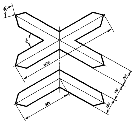
Рисунок Д.2. Размеры знаков 1.3.1 , 1.3.2
