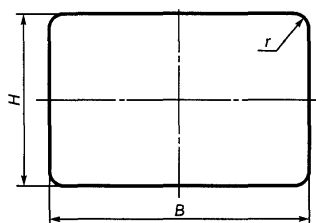
Рисунок Д.8. Размеры прямоугольных знаков горизонтального формата
