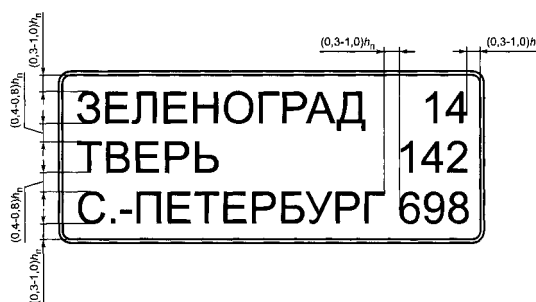
Рисунок Г.5. Пример компоновки знака индивидуального проектирования 6.12
