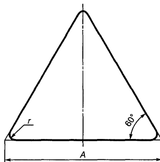
Рисунок Д.1. Размеры треугольных знаков
